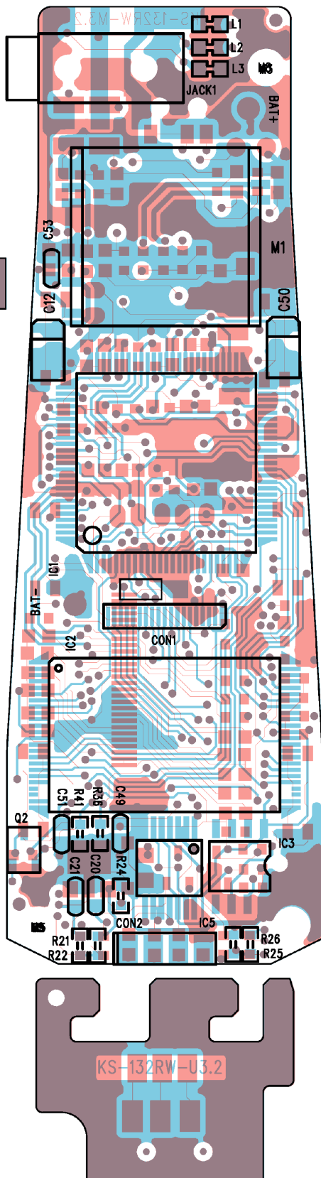
Layer 1 + 4
